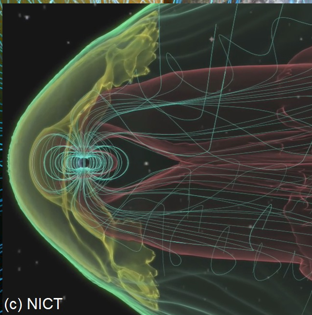
地球磁気圏
